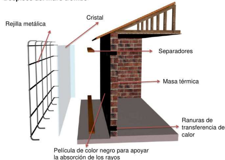
Despiece del muro trombe
